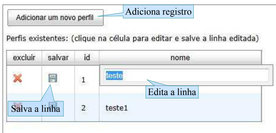
Ilustração 22: Uso do editor de tabelas auxiliares
